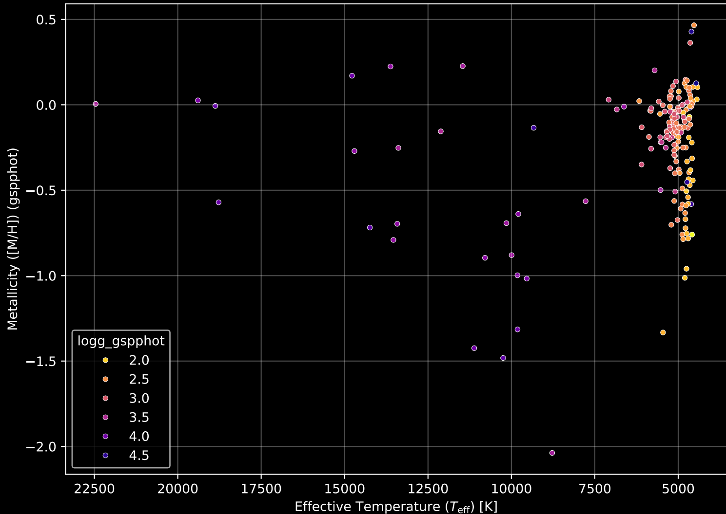
APOGEE DR17 Field: [COROTA] Stellar Population Parameters (n= 187)
